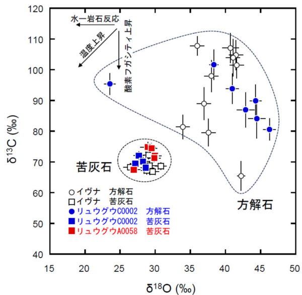
図2：リュウグウ試料およびイヴナ隕石中の方解石、苦灰石の炭素・酸素同位体比。方解石は苦灰石に比べて大きな変動を示す。水-岩石反応、温度上昇、酸素フガシィ上昇に伴う同位体比の変化は矢印で模式的に示す。
