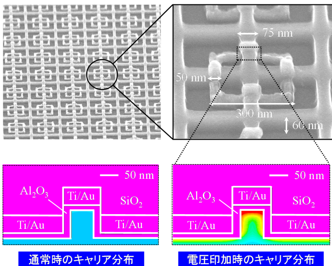
図2 電圧制御が可能なトライゲートメタマテリアル
