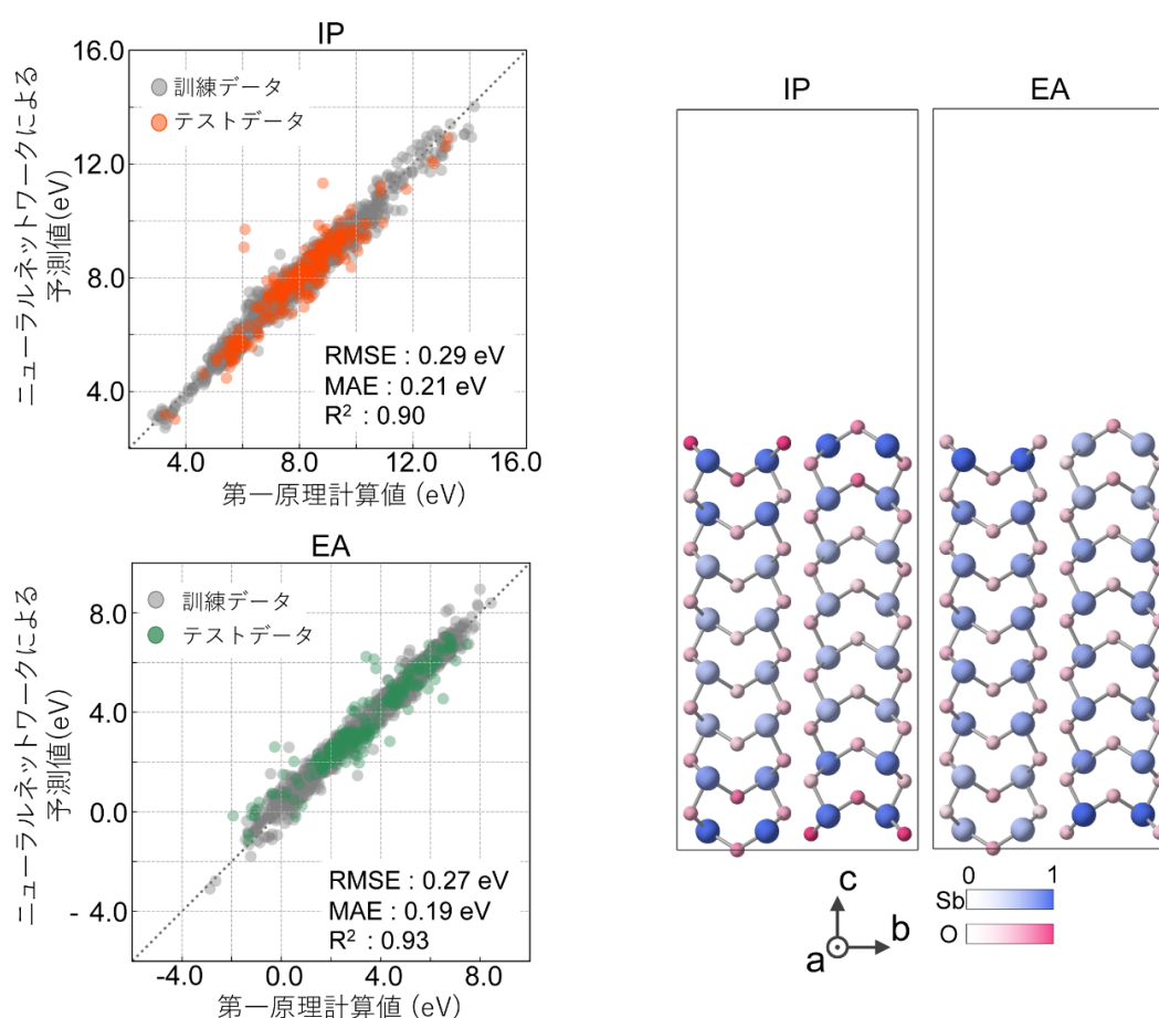
図 3 ニューラルネットワークを用いた二元系酸化物の IP・EA の予測 (左)。図中に 二乗平均平方根誤差 (Root-Mean-Square Error: RMSE) 、 平均絶対誤差 (Mean Absolute Error: MAE) 、 決定係数 (R 2 ) (用語 12) の値を示す。表面モデル内の各原子の IP・EA への影響の大きさ (右)。 \text{Sb}_2\text{O}_3 の(001)表面の例であり、色が濃いほど影響が大きいことを表している。
