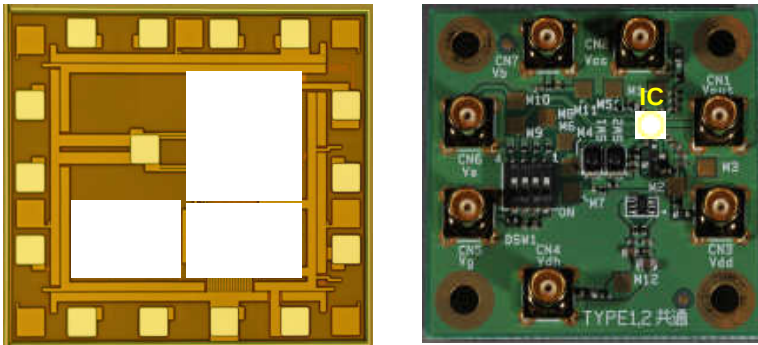
図6 (左) ICの顕微鏡写真。面積は、 1.4 \text{ mm}^2 である。 (右) ICを搭載した評価ボード。ICは帯域を確保するためにワイヤーボンディングではなくフリップチッププロセスによって評価ボードと接続した。
