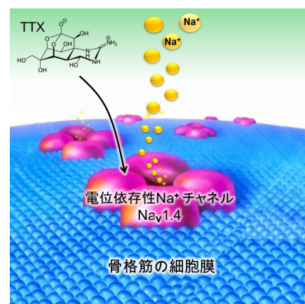
⑤ テトロドトキシン（TTX）の標的となる骨格筋の Na^+ チャンネル（実際には \alpha\beta サブユニットからなるが、ここでは \alpha のみ表示； \alpha は 4 つの類似ドメインからなり、中央部の穴が Na^+ の通路となる）。◆ 神経細胞からの情報を受け取ると骨格筋細胞は電位変化を起こす。この変化が電位依存性 Na^+ チャンネル（ Na_v1.4 ）によって検出・増幅されて、骨格筋の収縮装置に伝わる。テトロドトキシンが Na_v1.4 に結合すると、 Na_v1.4 の中央部のチャンネルが閉じたままとなり、収縮装置に情報が伝わらなくなる。バイオ系の学生のためにもう少し詳しく記すと次のようになる：
