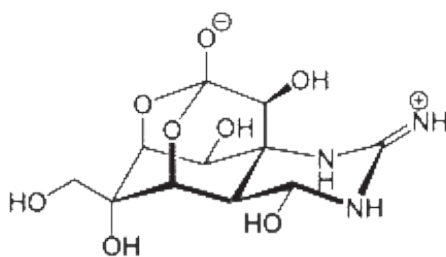
④ フグ毒（ C_{11}H_{17}N_3O_8 、テトロドトキシン、Tetrodotoxin, TTX）。1964 年 4 月、京都で第 3 回 IUPAC 国際天然物化学会議（The Third IUPAC Symposium on the Chemistry of Natural Products）が開かれ、Woodward ら（Harvard 大学）、津田ら（東京大学・三共）、後藤ら（名古屋大学）の 3 グループによりフグ毒 Tetrodotoxin の構造決定が同時に発表された（ 注13～15 ）。X 線構造解析による絶対配置の決定は 1970 年（ 注16 ）。ラセミ体の全合成は 1972 年に岸ら（ 注17 ）（名古屋大学、後に Harvard 大学教授）によってなされ、最終的な不斉全合成は、2003 年に達成された。（ 注18 ）
