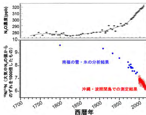
図2. 大気中N 2 Oの濃度と窒素同位体比の経年変化。(濃度は、中澤ほか「地球環境システム」共立出版(2015)による)
