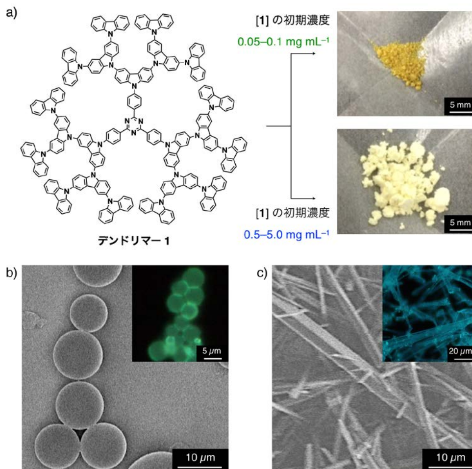
図 1. (a) コアにトリアジン、シェルに第 3 世代カルバゾールデンドロンをもつ \pi 共役デンドリマー 1 の分子構造、および 1 の初期濃度が異なるクロロホルム溶液に対しアセトニトリル蒸気を拡散することで得られる粉末の写真。(b, c) 初期濃度 0.1 mg/mL および 1.0 mg/mL の溶媒条件からそれぞれ生成したマイクロ球体 (b) およびマイクロファイバー (c) の電子顕微鏡写真と蛍光顕微鏡写真 (内挿図)。
