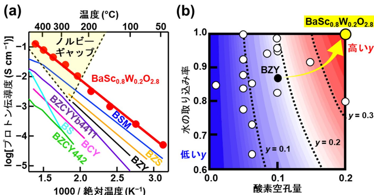
図 1 (a) \text{BaSc}_{0.8}\text{W}_{0.2}\text{O}_{2.8} と代表的なプロトン伝導体のプロトン伝導度の比較。(b) \text{BaSc}_{0.8}\text{W}_{0.2}\text{O}_{2.8} と代表的なプロトン伝導体の酸素空孔量、水の取り込み率とプロトン濃度 y の比較。(© Royal Society of Chemistry)
