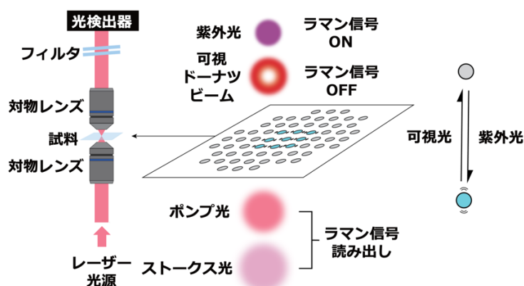
図 1：ラマンプローブによる超解像イメージング (RESORT) 法の模式図
