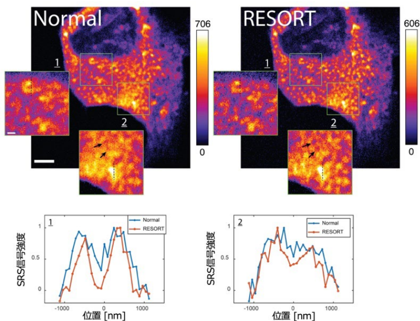
図 2 : (上) 細胞内ミトコンドリアの RESORT 画像。(下) 画像中の点線部のクロスセクション。
