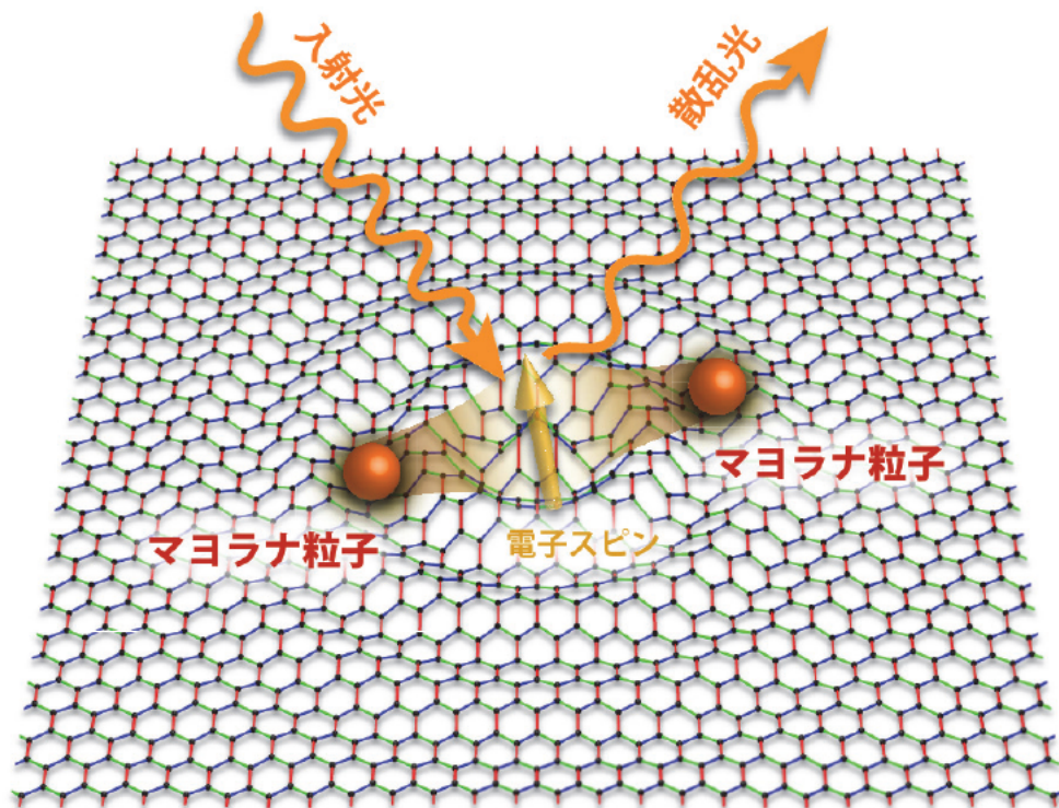
図 2 磁気ラマン散乱によるマヨラナ粒子創発の概念図。光の散乱によって電子スピンの分極化したマヨラナ粒子を 2 つ生成する。この過程が散乱強度の温度変化に現れる。
