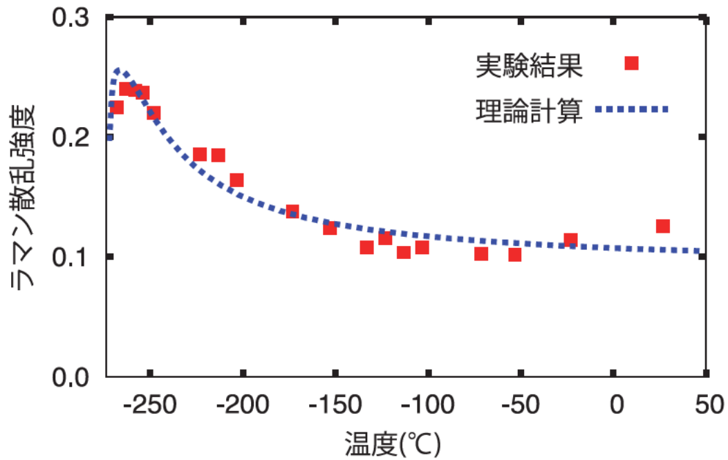
図 1 磁気ラマン散乱強度の温度依存性。塩化ルテニウムに対する実験結果と本研究でキタエフ模型に対して得られた理論計算結果との比較を示している。
