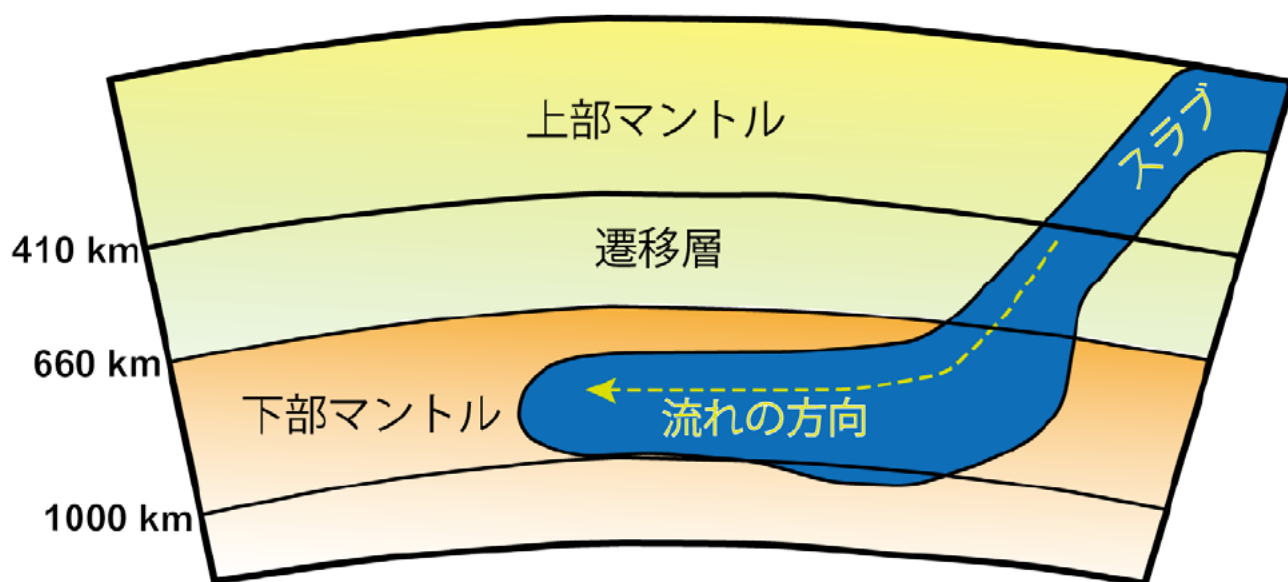
図 2. トンガ・ケルマディックスラブ近傍の地球マントルの内部構造
