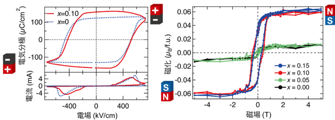
図2：室温における鉄酸ビスマスとコバルト酸鉄酸ビスマス（ x はコバルトの置換量）の電気分極の外部電場依存性（左）および磁化の外部磁場依存性。
