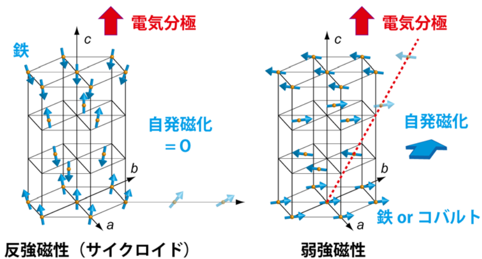
図1：鉄酸ビスマス（左）とコバルト酸鉄酸ビスマス（右）の磁気構造の模式図。鉄酸ビスマスは反強磁性体であるため、スピンの磁化は打ち消し合い自発磁化は現れない。一方、コバルト酸鉄酸ビスマスはスピンの傾斜しているため、磁化は打ち消し合わずに自発磁化が現れる。
