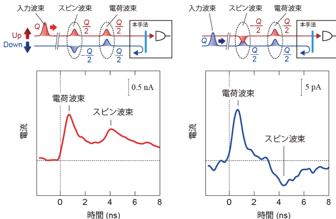
図2: スピン電荷分離現象の測定例 (左) アップスピン電子集団 (波束) 入力時の測定結果 (右) ダウンスピン電子集団 (波束) 入力時の測定結果
