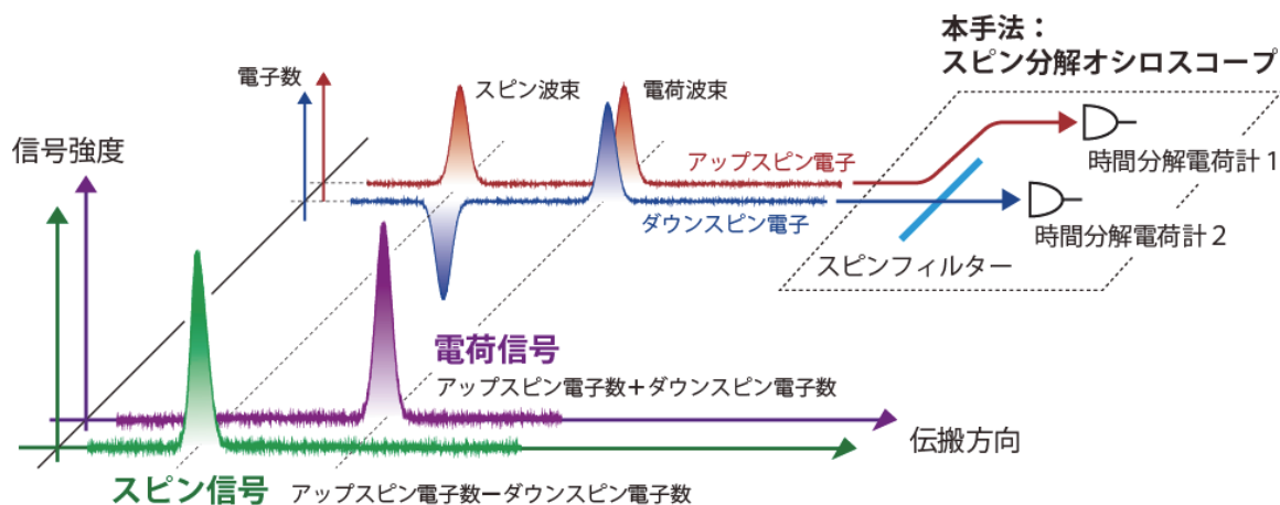
図1：スピン分解オシロスコープによる電荷信号・スピン信号測定概念図
