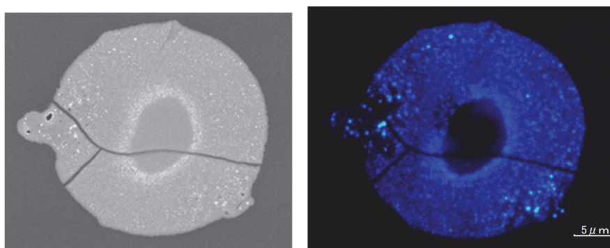
図 1 ナノコンポジット蛍光体断面 SEM 像（左）と電子線発光像（右）
