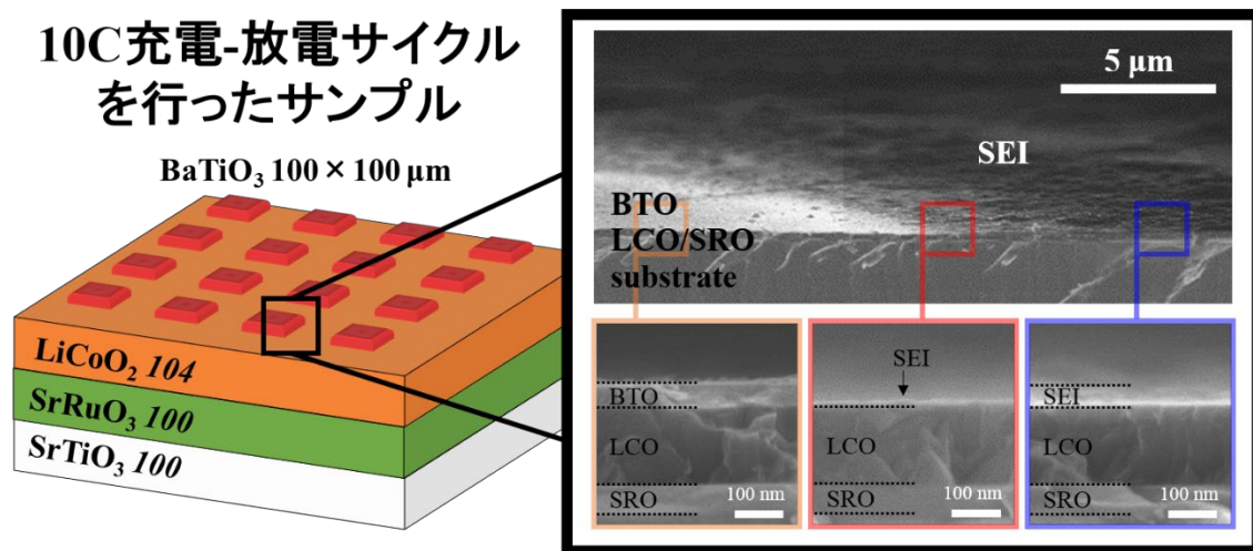
図2 LCO表面に100 μm角のBTOを堆積させた薄膜の模式図（左図）と、10Cにて充電／放電を行った後の走査型電子顕微鏡観察像（右図）。
