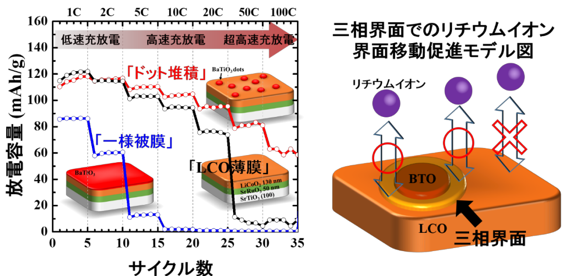
図1 今回作製した3種類の薄膜（LCO薄膜：黒線、一様被膜：青線、ドット堆積：赤線）の段階的にCレートを増加させて充放電を行った際の放電容量の変化（左図）。また、今回判明した三相界面でリチウムイオンの界面移動が促進されているモデル図（右図）。
