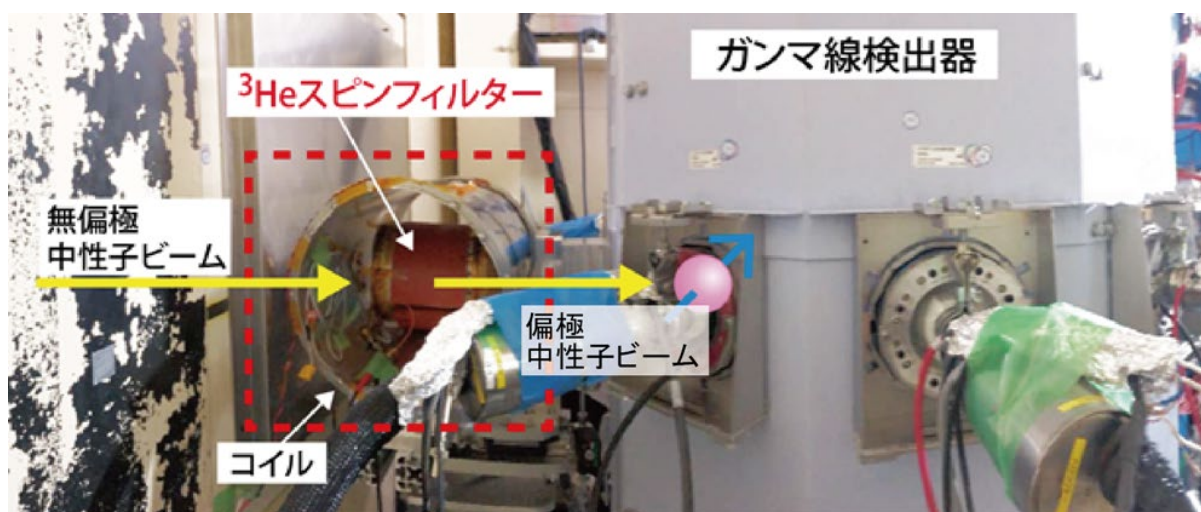
図1 ガンマ線検出器の上流に設置した偏極装置( ^3\text{He} スピンフィルター)
