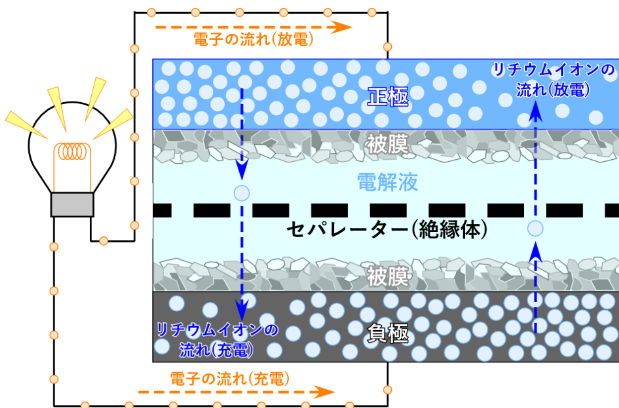
図 1: リチウムイオン電池の模式図
