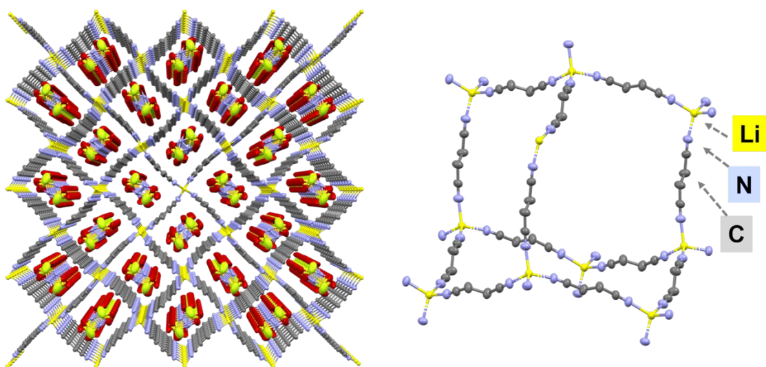
図3．単結晶 X 線構造解析で明らかにした \text{Li(FSA)(SN)}_2 の結晶構造（左）パッキング図、（右）Li イオンと SN で形成されるダイヤモンド状構造（FSA アニオンは省略）
