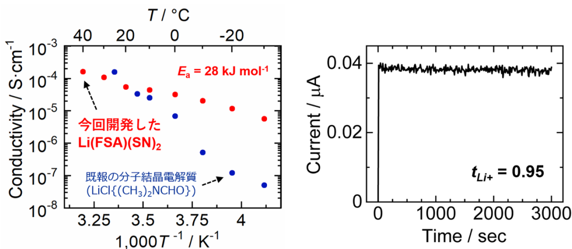
図4． \text{Li(FSA)(SN)}_2 の結晶状態におけるイオン伝導度（左）とリチウムイオン輸率測定（右）の結果
