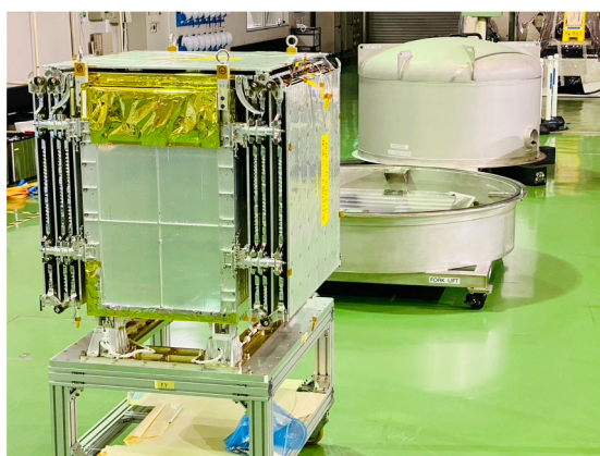
出荷直前、コンテナ納入前の"StriX-a"
