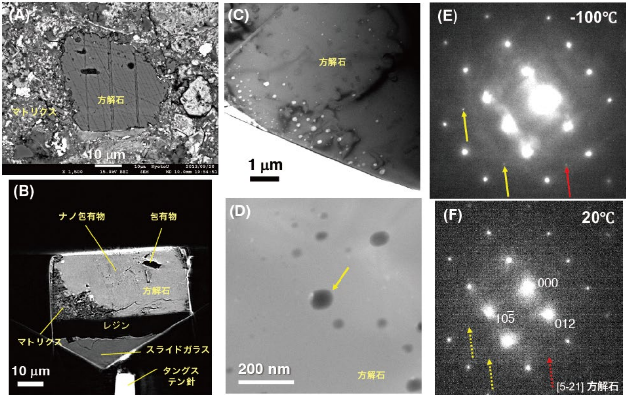
図1 サッターズミル隕石の鉱物中の CO 2 に富む流体包有物の発見。(A) 隕石の走査型電子顕微鏡 (SEM) 写真。方解石 (CaCO 3 ) と呼ばれる鉱物に着目した。(B) サンプルの X 線ナノ CT 像。FIB を用いて方解石を含む領域を切り出し、SPring-8 において X 線ナノ CT 撮影を行った。数ミクロンの比較的大きな包有物だけでなく、ナノサイズの包有物も多数存在することがわかった。(C) 方解石中のナノ包有物の透過型電子顕微鏡 (TEM) 像。ナノ包有物が多数存在する領域を、イオンビームを用いて薄く切り出し、TEM 観察を行った。(D) CO 2 に富む流体包有物を含むナノ包有物 (黄色の矢印の先) の TEM 像。(E, F) (D) の包有物を含む領域の電子線回折図形。明るい斑点は方解石の回折によるもの。-100°C で見えている余分な斑点 (E: 黄色の矢印の先) の位置とこれらが 20°C では消える (F) ことから、CO 2 と H 2 O の化合物あるいは CO 2 の氷の存在がわかった。
