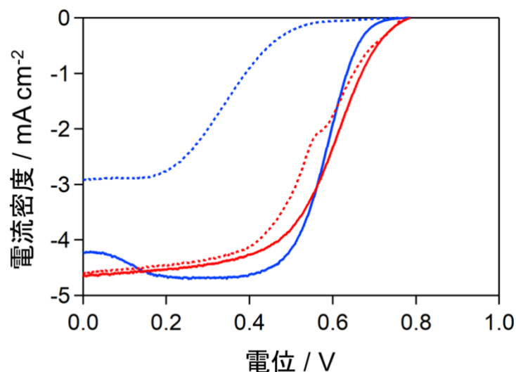
図2 電位掃引試験前後(実線が前、点線が後)の触媒活性の比較。高い電位(横軸右方向)で大きなマイナス電流(縦軸下方向)を示す触媒が高活性。鉄フタロシアニン(青)は劣化が著しいが新物質(赤)は優れた触媒活性を持続する。
