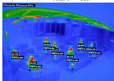
▲実証実験イメージ 熱画像センサーと AI を利用した快適性の見える化
