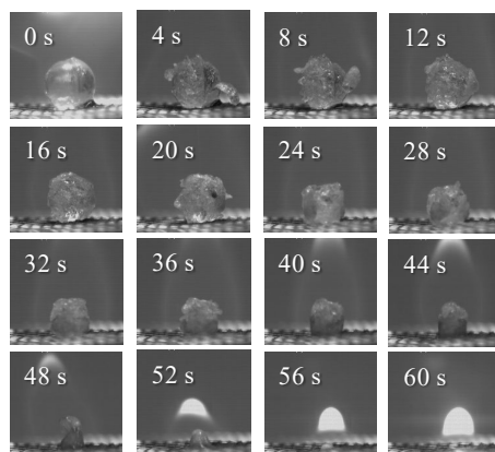
図 2. エタノールを含有した高分子ゲルの燃焼の様子
