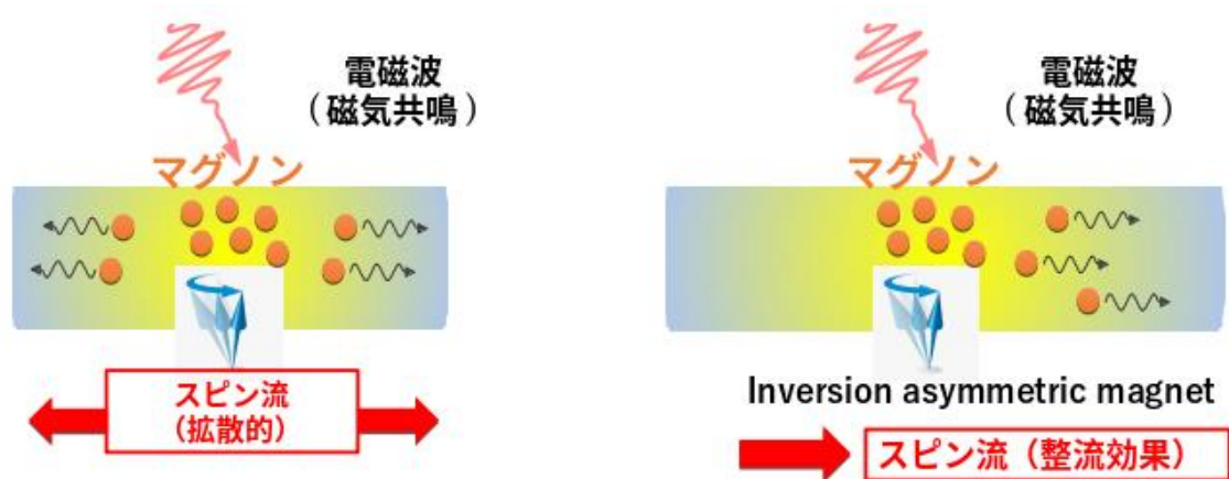
図 2：スピンプンプによる拡散的スピン流（左）と整流効果によるスピン流（右）。
