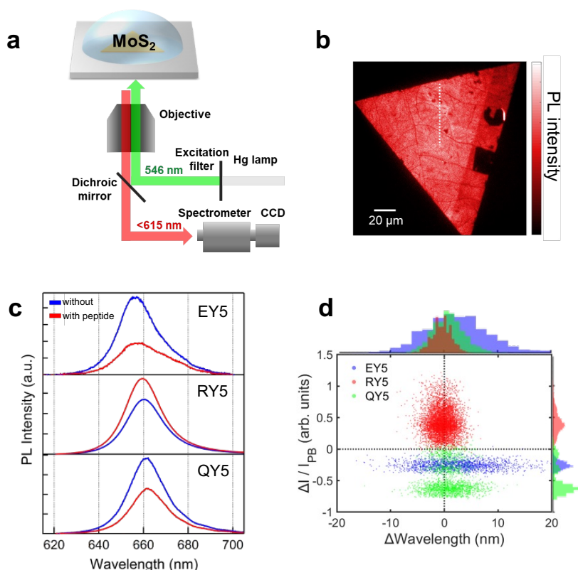
図 4： (a) \text{MoS}_2 の発光測定システムの模式図。(b) 単層 \text{MoS}_2 の発光イメージ。(c) \text{MoS}_2 の発光スペクトル。青色と赤色の曲線はそれぞれ、ペプチドの修飾前と後のスペクトルを示す。(d) 発光ピークの強度の変化量（縦軸）とピーク波長の変化（横軸）をそれぞれのペプチドで散布図にしたもの。
