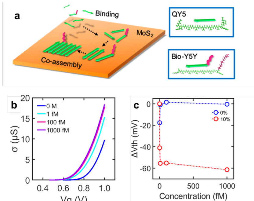
図5：(a) ビオチン化ペプチドと足場ペプチドの共自己組織化の模式図。(b) MoS 2 トランジスタのタンパク質濃度に応答した変化。(c) トランジスタの閾値電圧の変化。ビオチン化ペプチドが全体のペプチドの10%含まれる場合(赤色)と含まれない場合(青色)の結果。
