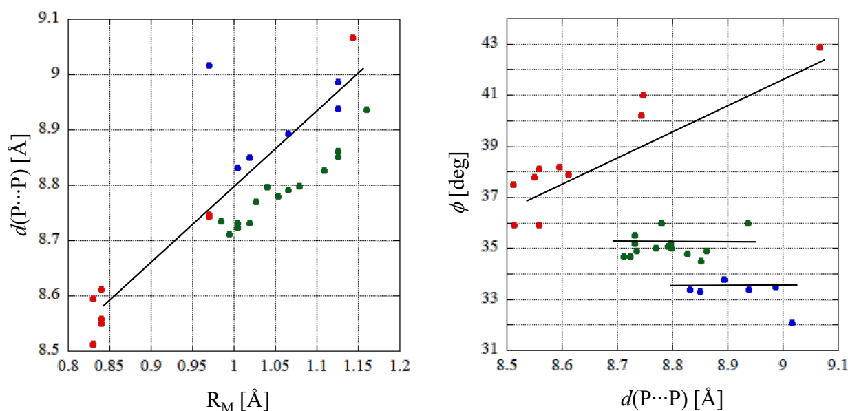
図 2: 各カチオン、共存物質別の、 R_M に対する d(P \cdots P) (左)、 d(P \cdots P) に対する \phi のプロット (右)。赤は、アンモニウム塩、青はアルカリ金属塩、緑は共存物質にプロリンを導入した化合物群。各カチオン別に分布があり、それぞれに傾向が現れているのが分かる。
