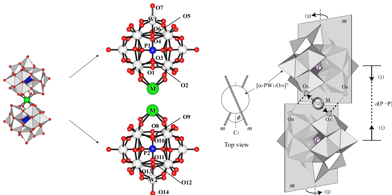
図 1. 幾何学的パラメータの設定。構造解析によって明らかになったポリ酸アニオンの構造から、 R_M 、 d(P \cdots P) 、 \phi 、 d(O_A \cdots O_{A'}) 、 \phi(\angle P-M-P) を設定した。 \phi を決める二面角 m は、骨格構造に示されている原子によって作られた。
