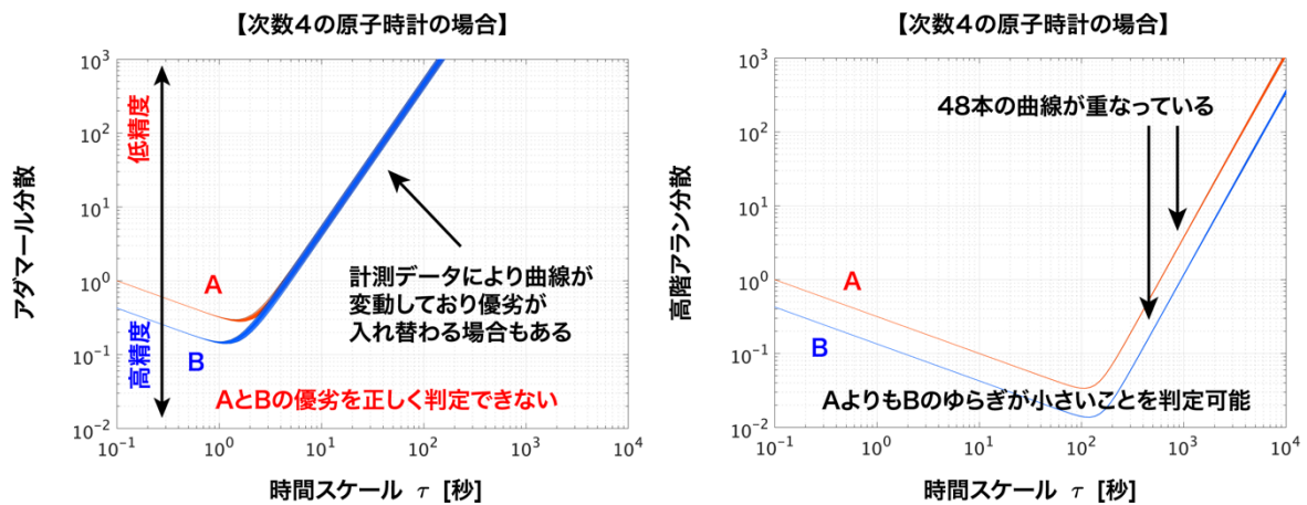
図3：次数4の原子時計に対するアダマル分散（左）と高階アラン分散（右）の曲線（原子時計AよりもBの時刻ゆらぎが小さい）
