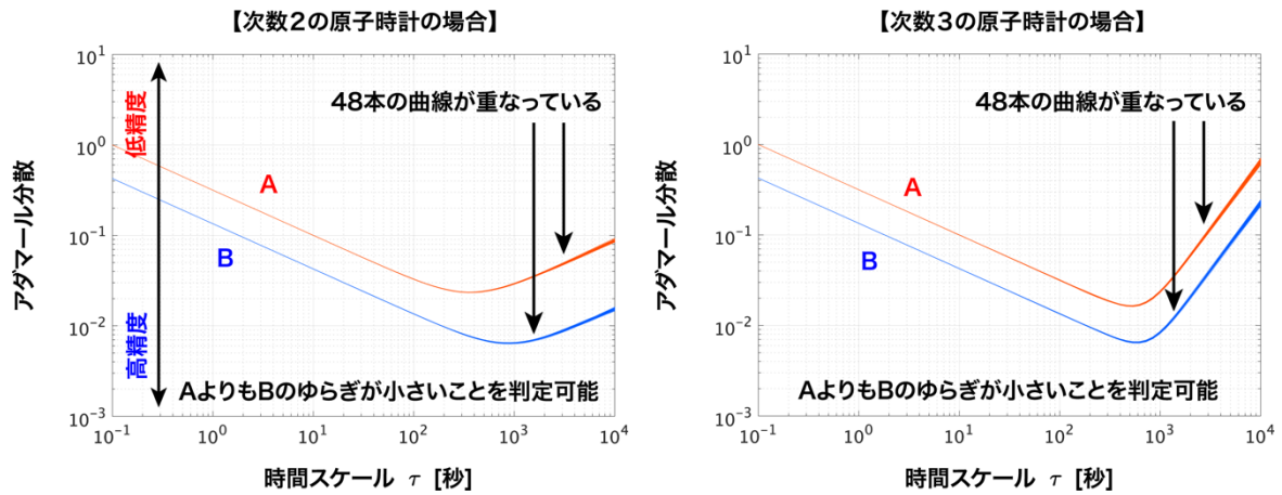
図2：次数2の原子時計（左）と次数3の原子時計（右）のアダマル分散の曲線（原子時計AよりもBの時刻ゆらぎが小さい）
