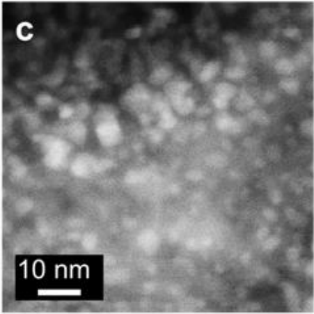
図 6. Ru/CaFH の電子顕微鏡写真
