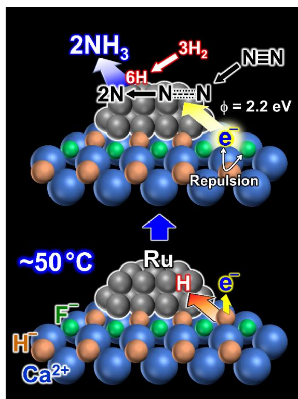
図 7 Ru/CaFHの予想メカニズム
