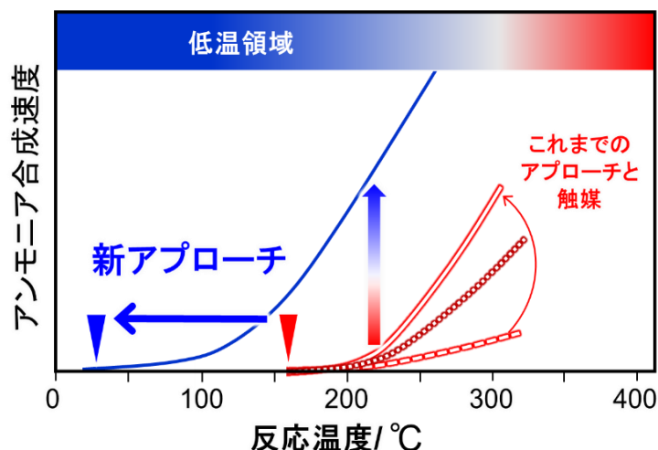
図3. アンモニア合成速度—反応温度曲線
