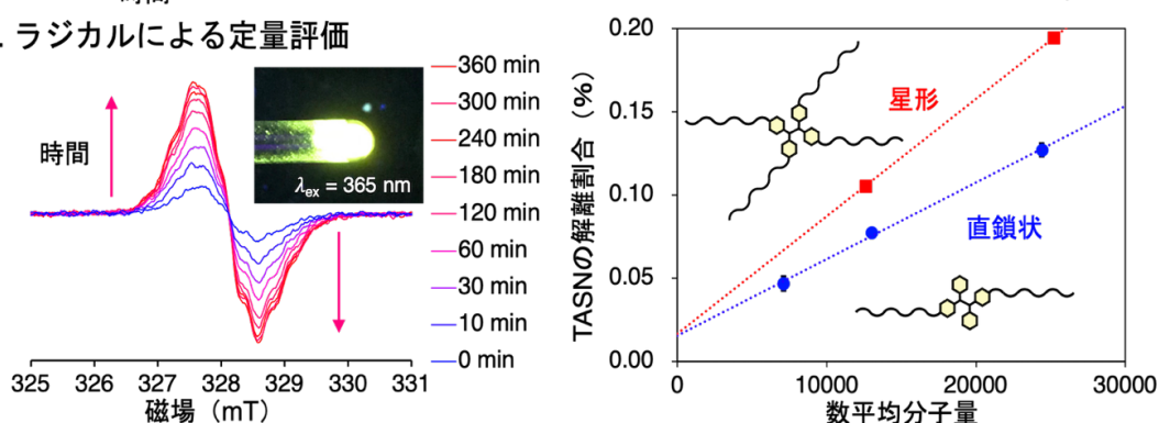
図 3. 力学応答分子を利用した結晶化誘起メカノフルオレッセンス（用語 10）
