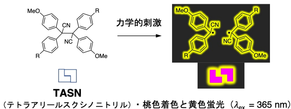
図 1. 本研究で使用した力学応答分子 (TASN) の化学構造と 力学的刺激によって発生する安定ラジカルの特徴
