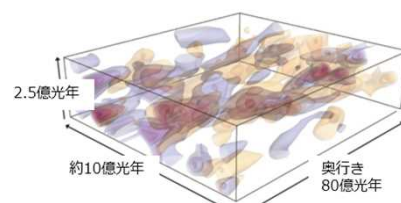
すばる望遠鏡が描き出した暗黒物質の三次元地図。宇宙での物質集積の歴史の一端が明らかになった。
