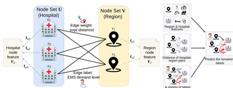
2部グラフ畳み込みニューラルネットワーク による救急医療サービスの予測
