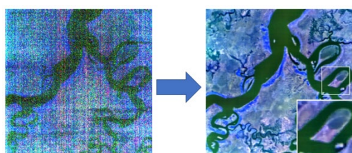
数理の力でセンシングデータから 価値ある情報を抽出
