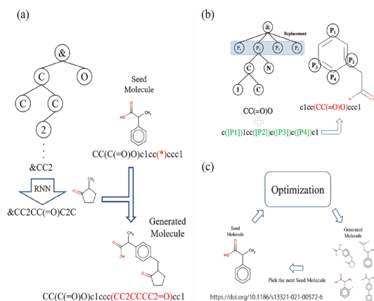
マテリアルズインフォマティクスによる分子設計
