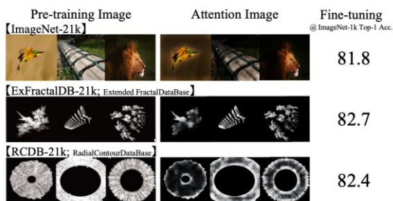
フラクタルを用いたVision Transformerの大規模事前学習
