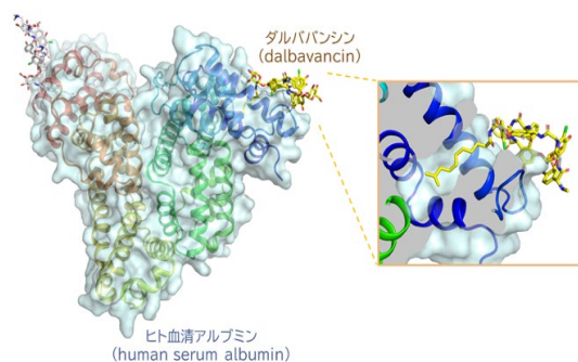
分子動力学計算によるタンパク質と薬分子のドッキングシミュレーション
