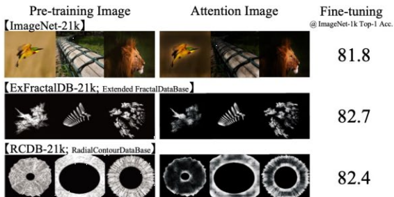
フラクタルを用いたVision Transformerの大規模事前学習
